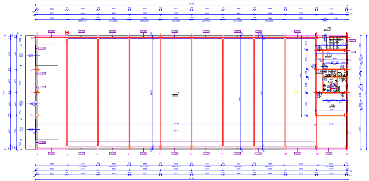
PÓDORYS 1NP M 1:100
